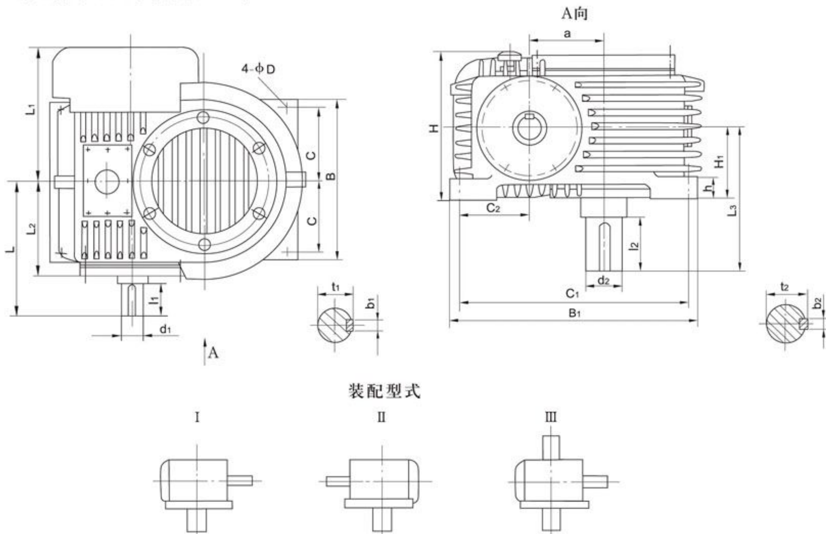
PWS 型减速器外形尺寸及装配型式
